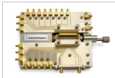
10GHz 通信用レーザー用
