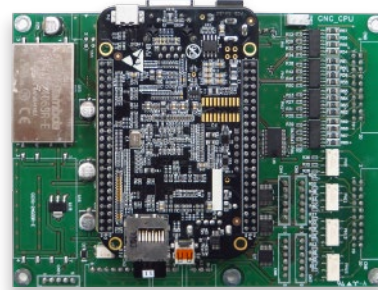
CPUボード
