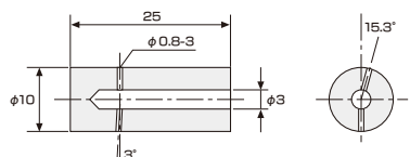
Φ0.8mmの穴加工が3箇所、 うち1つが3度の斜め穴加工を施しています。
